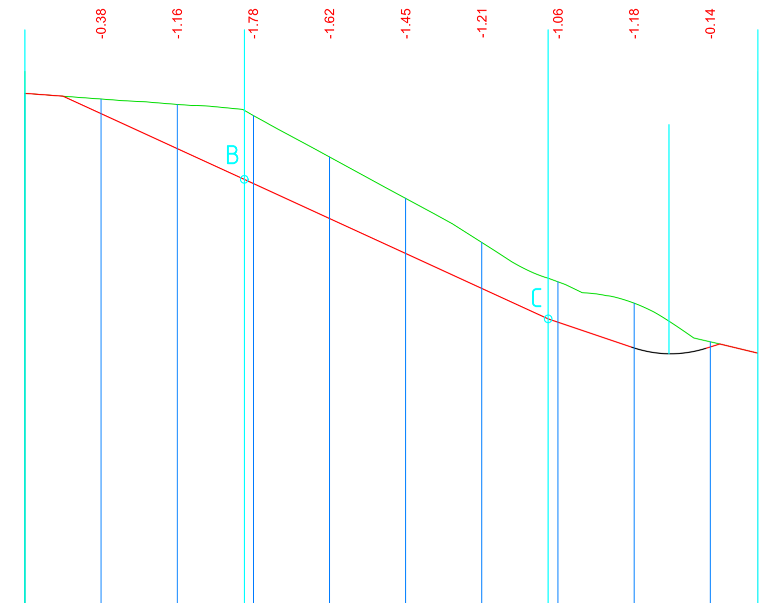
М 1:1000 по горизонтали М 1:100 по вертикали
